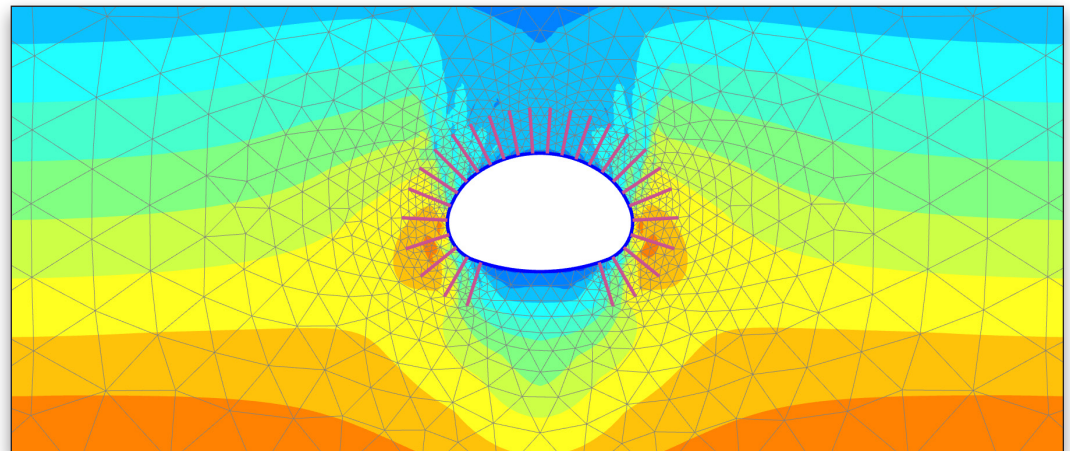
NATM-Tunnel mit Gebirgsankern.
